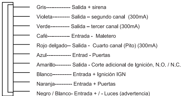
Conector de 10 pines
