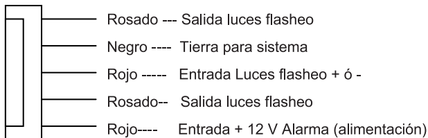
Conector de 5 pines
